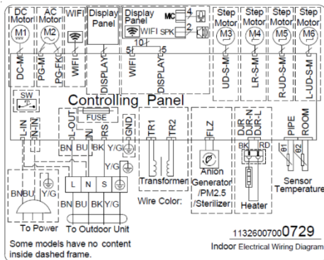
Рис. 23 Электрическая схема для внутренних блоков мощностью 9 000, 12 000, 18 000, 24 000 BTU, переводы см. таблицы 9-10.
