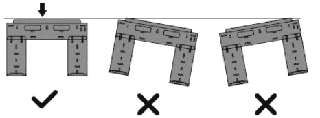
Рис.6 Правильное расположение монтажной пластины
