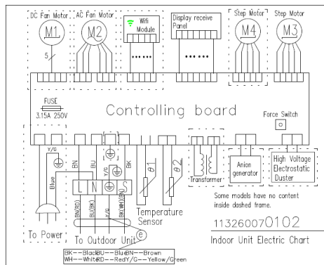
Рис. 22 Электрическая схема для внутренних блоков мощностью 7 000 BTU, переводы см. таблицы 9-10.
