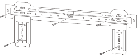
Рис.5 Монтажная пластина
