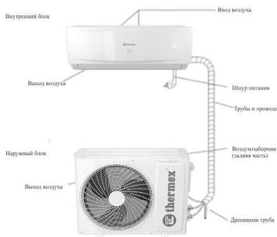
Рис.1 Расположение элементов сплит-системы
