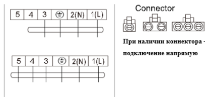
Рис. 20 Подключение внутреннего блока. Данная инструкция включает себя общие схемы на разные типы кондиционеров Thermex.
