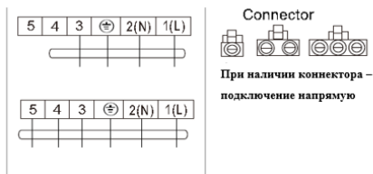
Рис. 20 Подключение внутреннего блока
