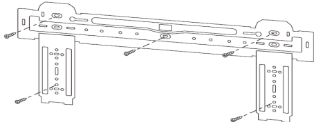
Рис.5 Монтажная пластина
