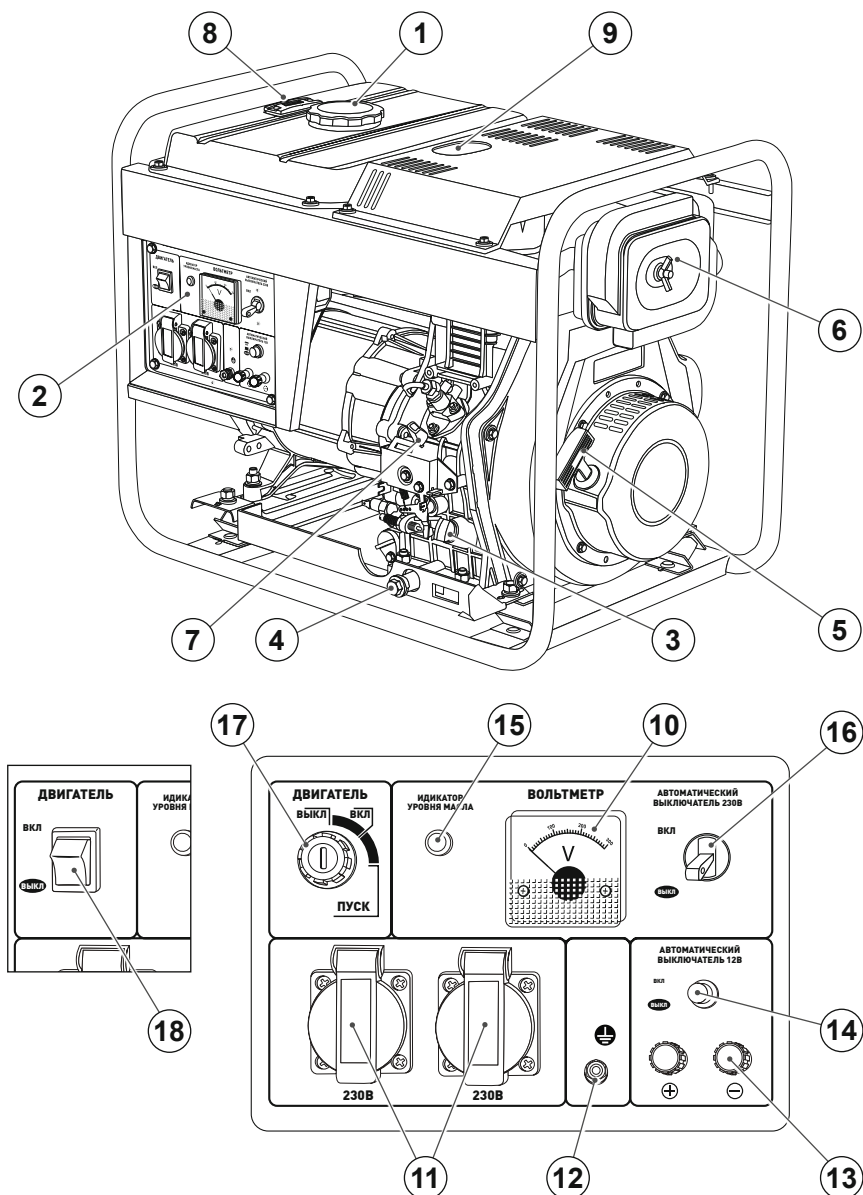
Рис. 1. Генератор
