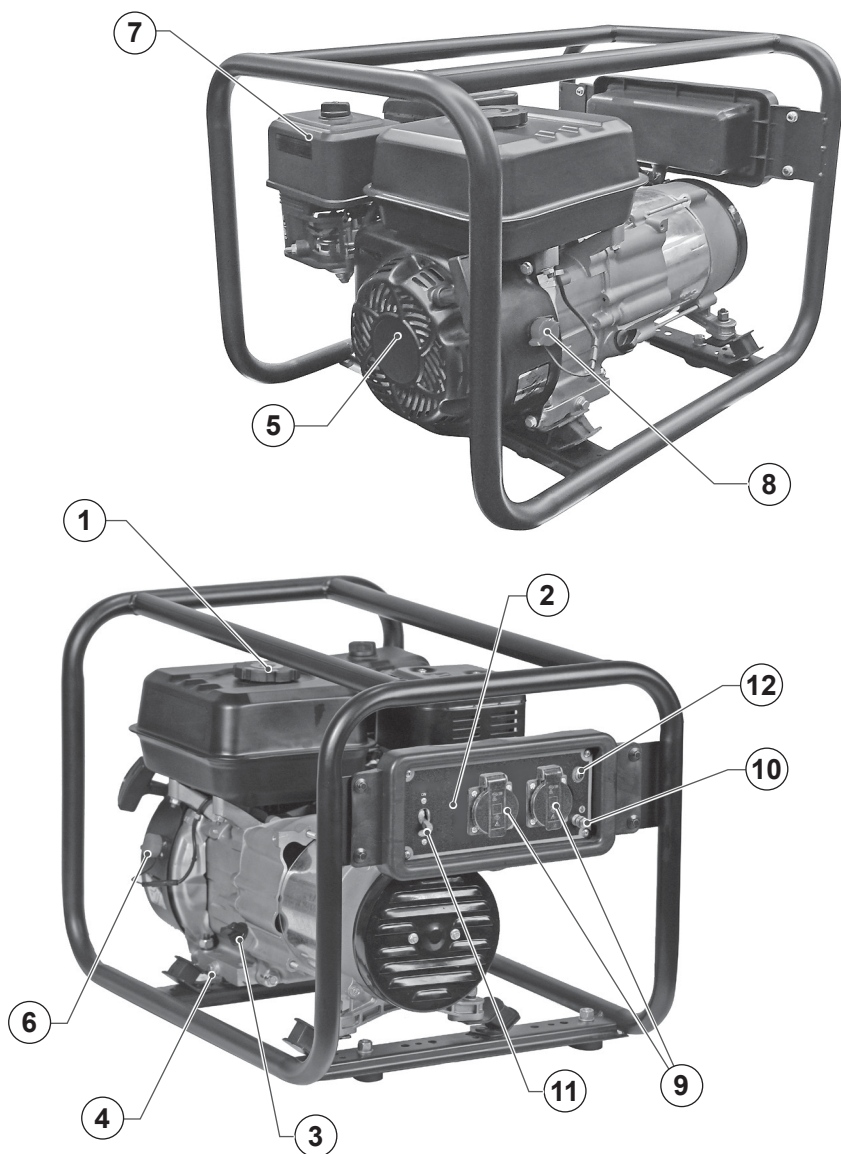
Рис. 1. Генератор
