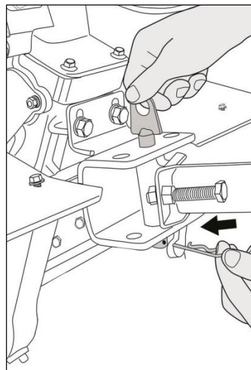
Рис.15 Фиксация пальца сцепки шплинтом
