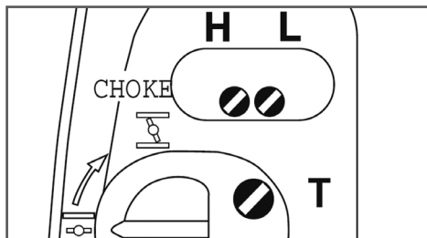
Рис. 24 Расположение винтов регулировки карбюратора
