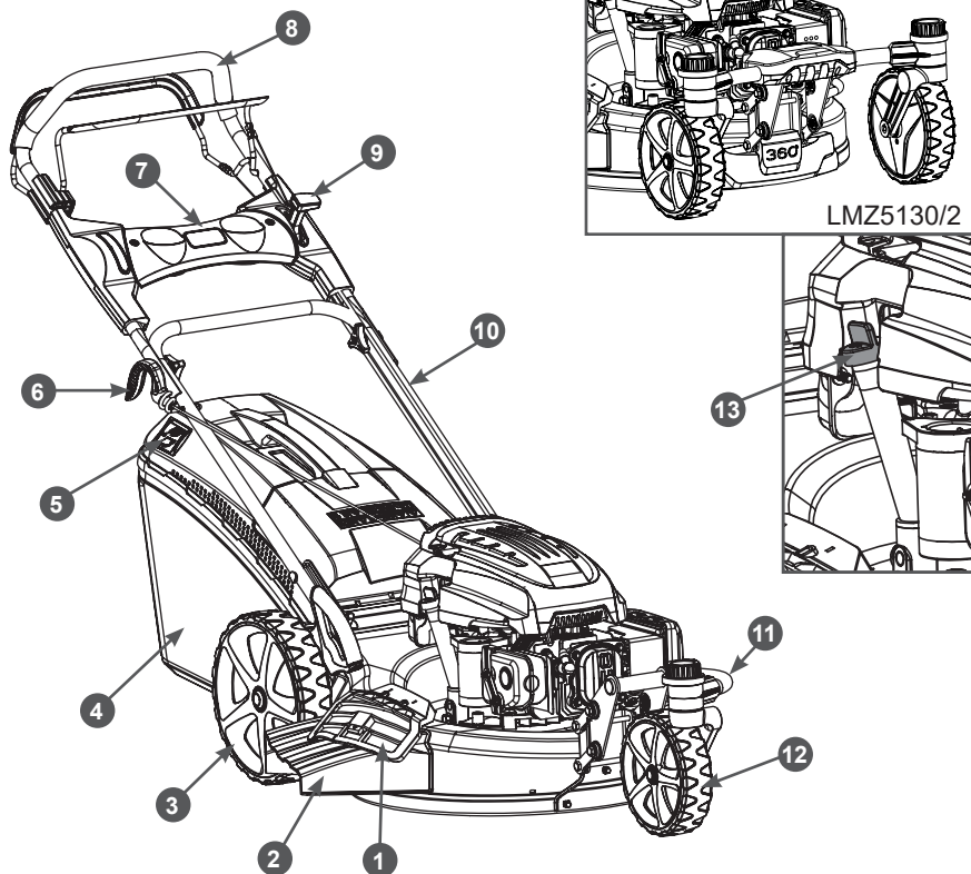
Рис. 1. Основные узлы и органы управления (вид справа)
