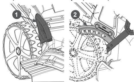
Рис. 18. Регулировка высоты скашивания
