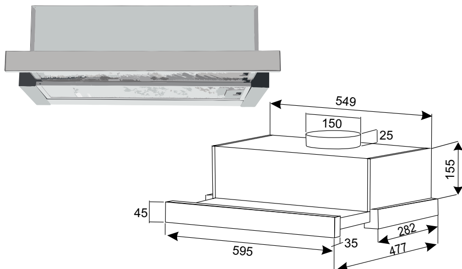
Рис. 1 Внешний вид кухонной вытяжки и схема размеров
