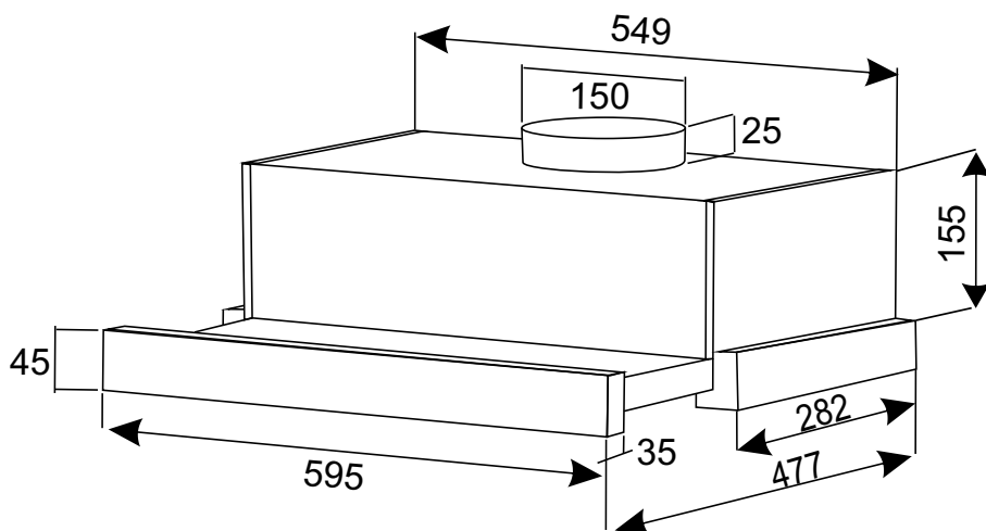
Рис. 8 Схема монтажа вытяжки
