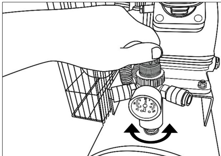
Рис. 11. Регулировка давления
