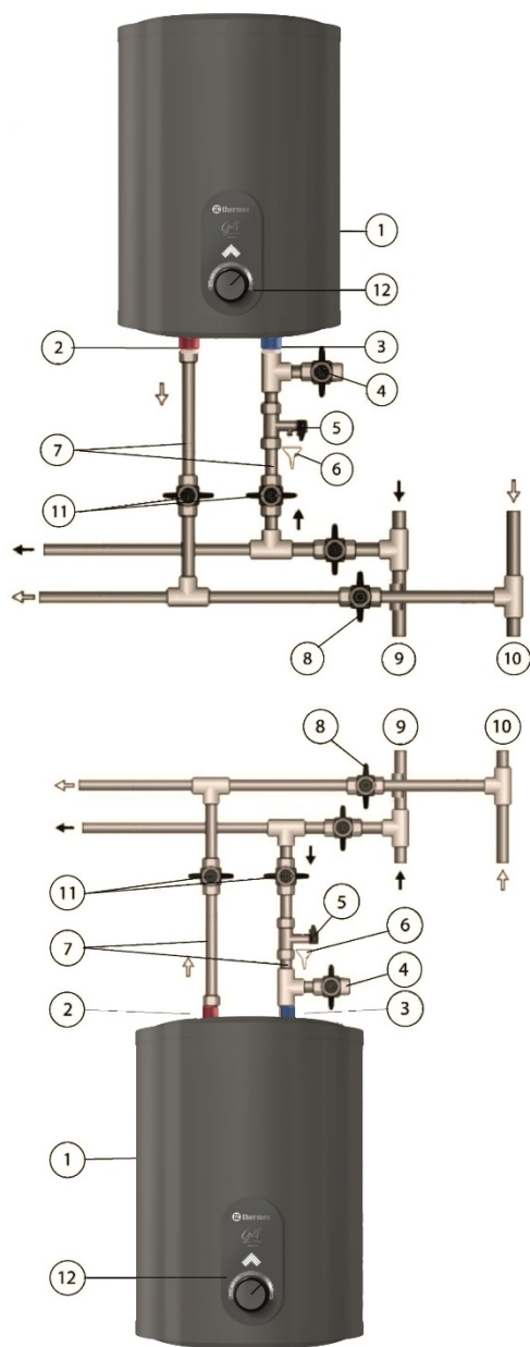
Рисунок 1. Схема подключения
