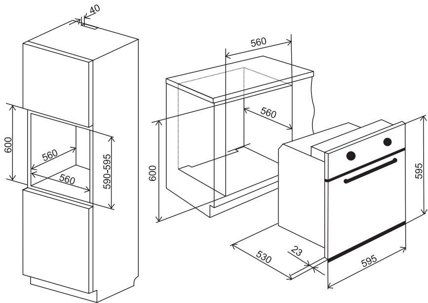
Схема встраивания
