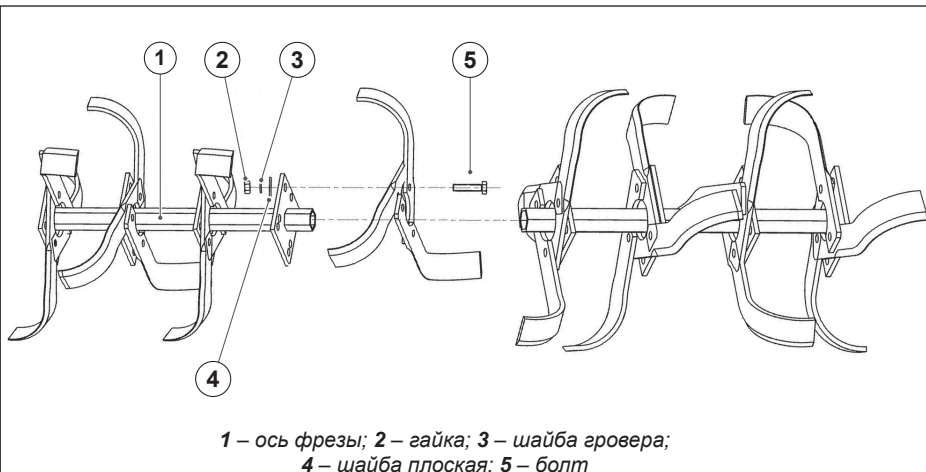
Рис. 4а. Сборка фрез с тремя ножами
