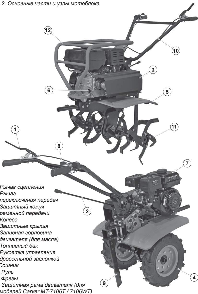
Рис. 2. Основные части и узлы мотоблока
