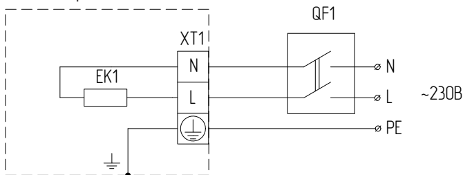
Рис. 3. Обогреватель ВИН-APL-1.5
