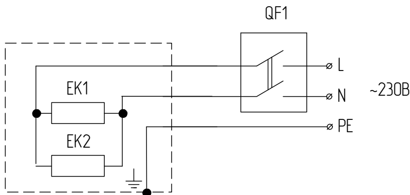
Рис. 1 Обогреватель для KIRH-E06P-11, KIRH-E08P-11, KIRH-E08P-12, KIRH-E10P-11, KIRH-E10P-12
