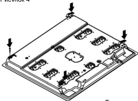
Точки крепления для фиксирующих зажимов
