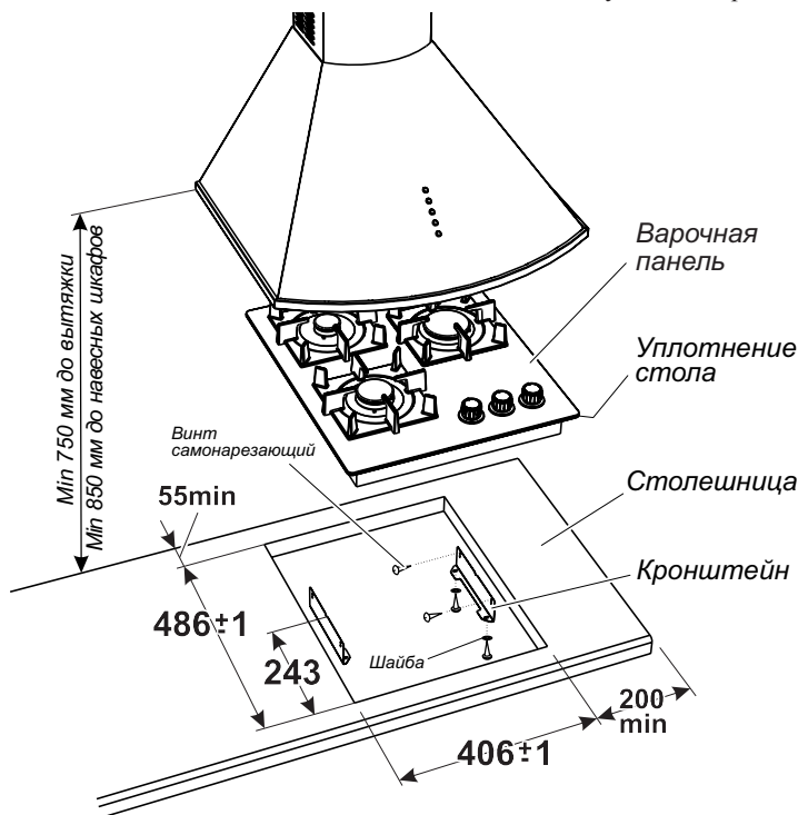
Рис. 9 МОДЕЛЬ ПВГ 2100; ПВГ 2100-01; ПВГ 2100-02
