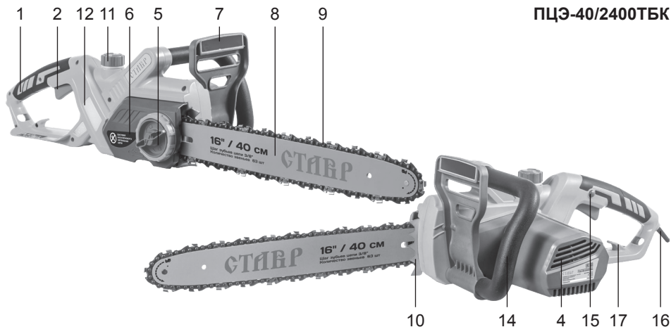
ПЦЭ-40/2400ТБК
