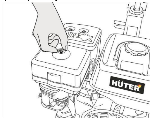
Рис. 37. Закрытие крышки воздушного фильтра
