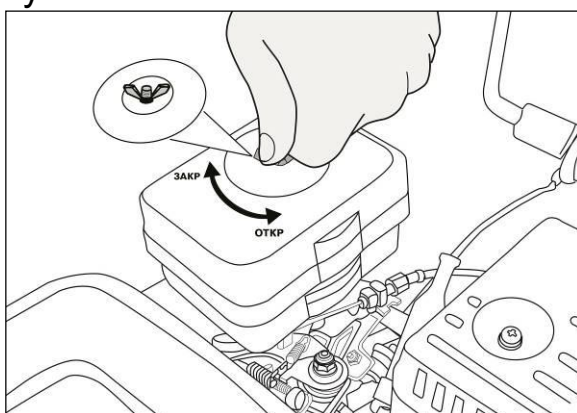
Рис. 24. Открытие крышки корпуса воздушного фильтра
