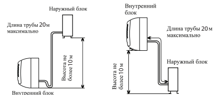
схема установки
