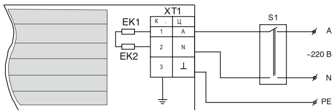
Рис. 2. Обогреватель RTI-20
