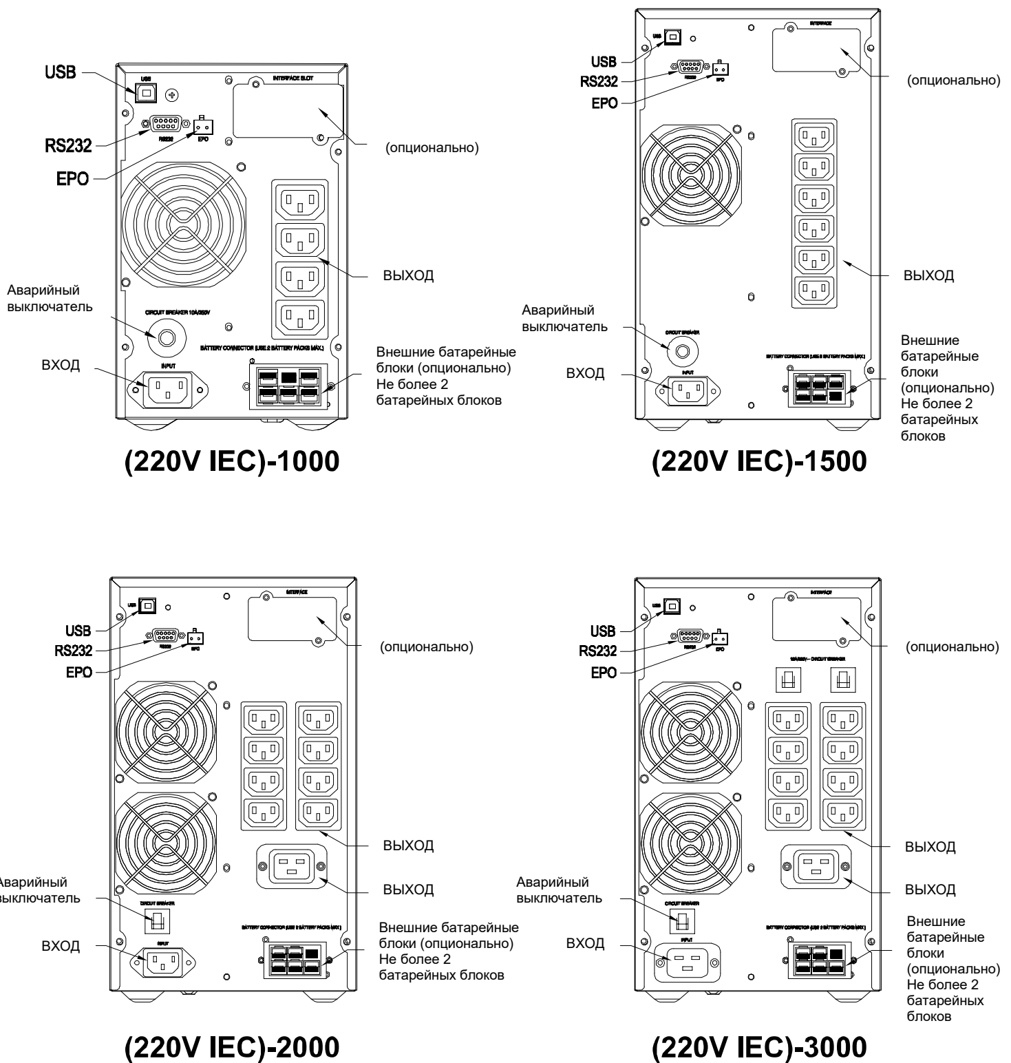
Рис. 4. Задняя панель серии MAC
