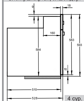
Электршкафтың өлшемдері
