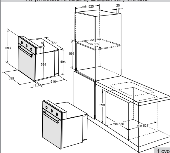
Электршкафтың өлшемдері
