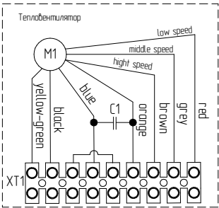
Внутренняя схема клеммной коробки тепловентилятора.
