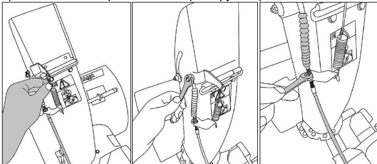
Рис. 18. Установка тросика
