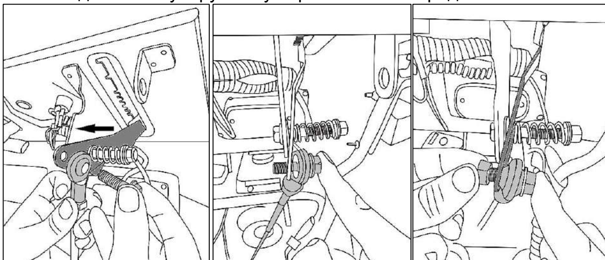
Рис. 14. Установка тяги
