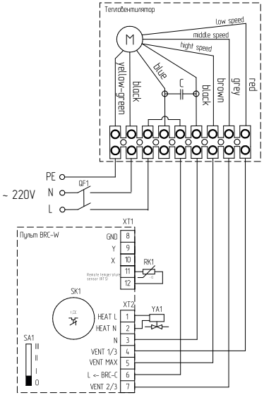
Подключение водяного тепловентилятора к пульту BRC-W.
