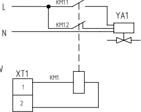
Схема подключения BRC-W
