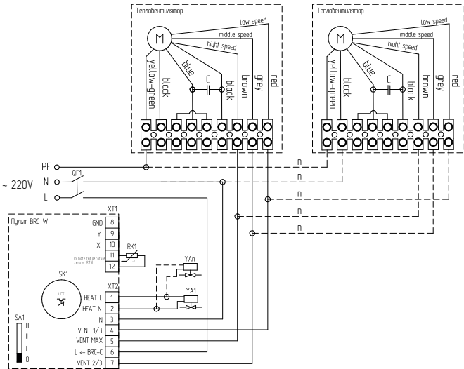
Групповое подключение водяных тепловентиляторов к пульту BRC-W.
