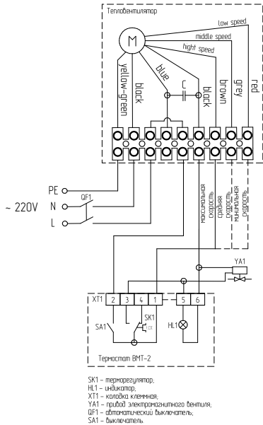
Групповое подключение водяных тепловентиляторов к термостату BMT-2, осуществление регулировки температуры воздуха, подачи теплоносителя.
