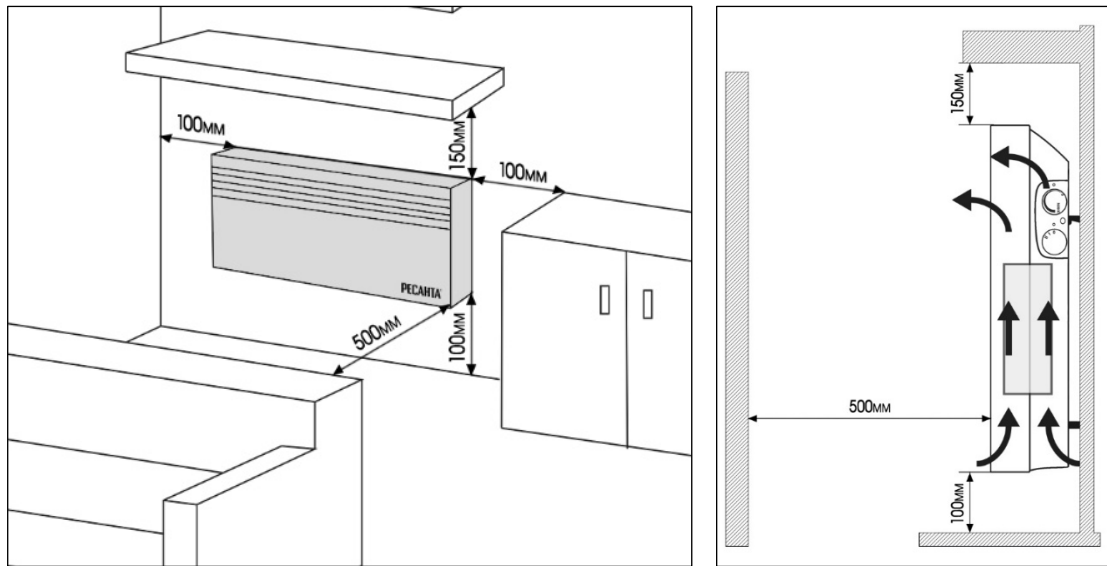
Рис. 3. Расположение конвектора.
