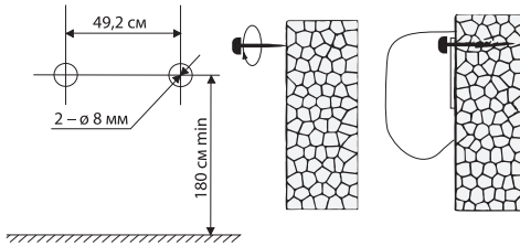
Мал.3. Схема установки приладу
