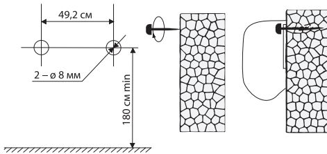
Рис. 4. Схема установки прибора
