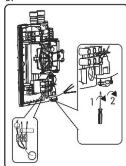
3-сүр. Thermex Surf 5000, Surf 6000 АЭСЖ құрастыру
